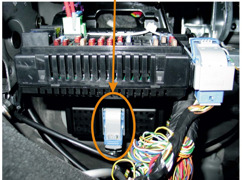
МОДУЛЬ СЕМ (над ногами водителя)
