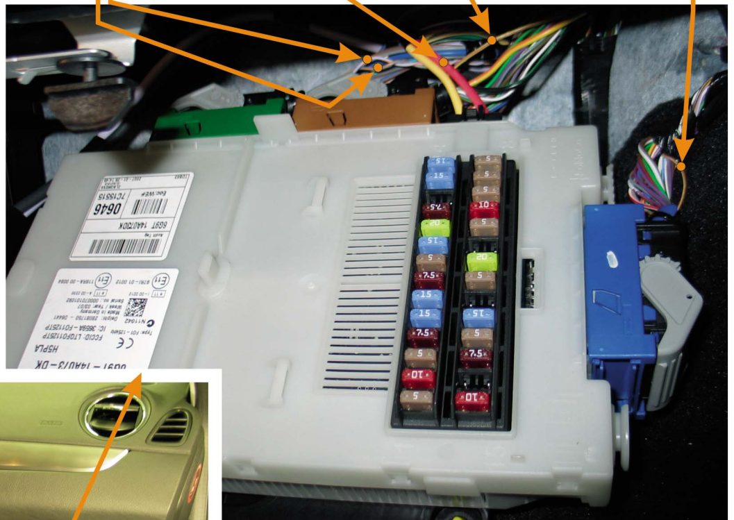
МОДУЛЬ (под перчаточным ящиком - сторона пассажира)
