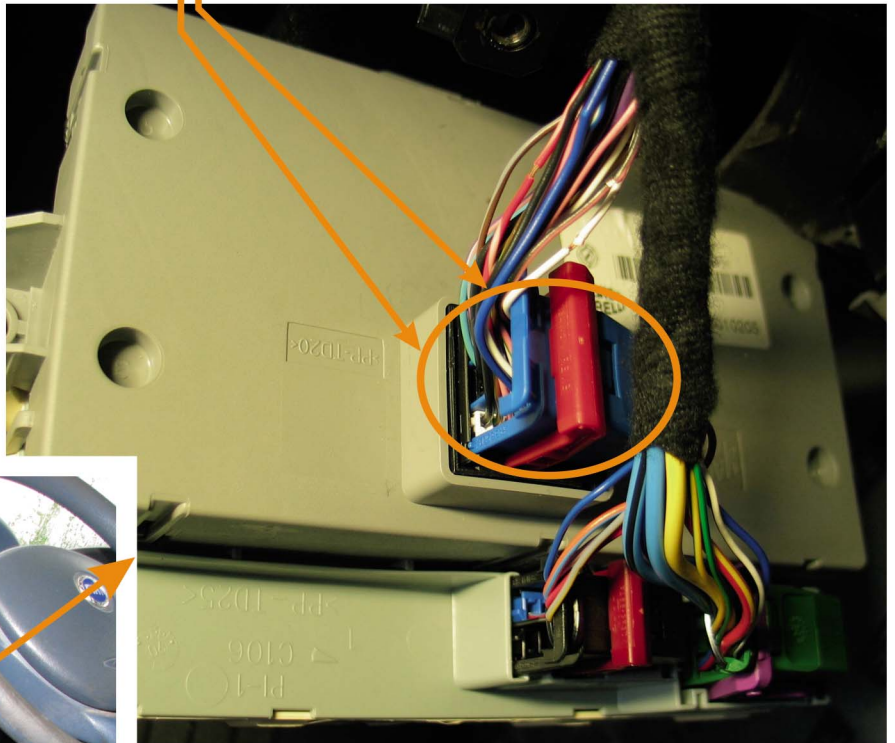
УПРАВЛЯЮЩИЙ МОДУЛЬ (ЗАДНЯЯ ЧАСТЬ)
