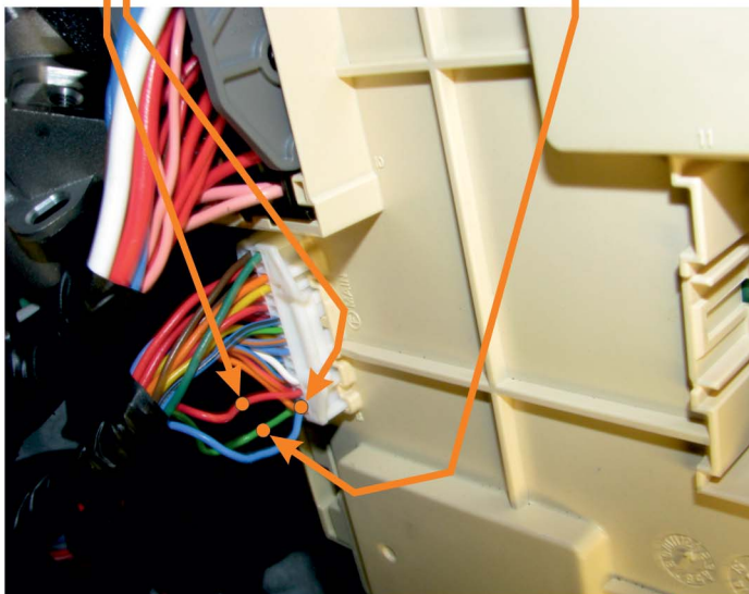
КОРОБКА ПРЕДОХРАНИТЕЛЕЙ (ЗАД)
