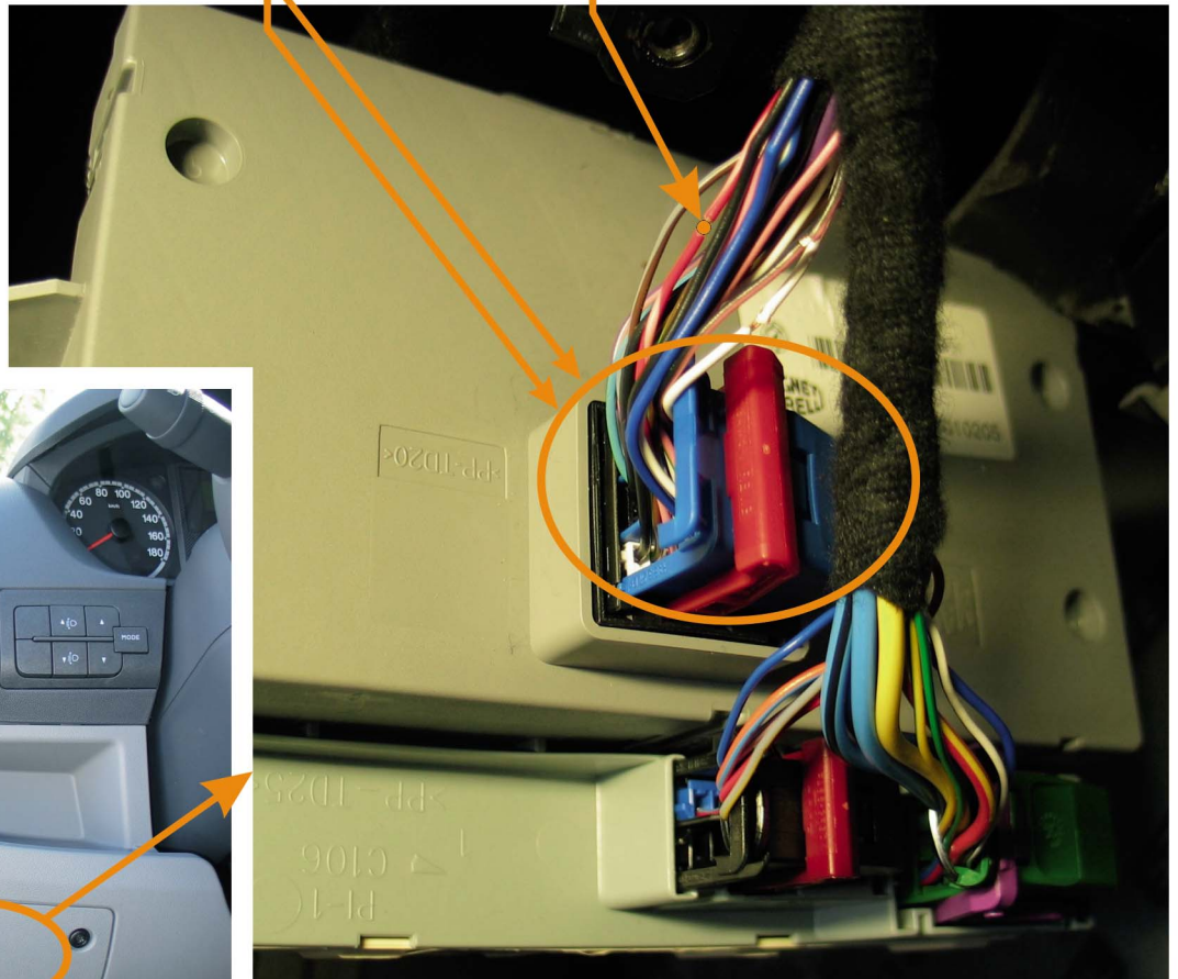
УПРАВЛЯЮЩИЙ МОДУЛЬ (ЗАДНЯЯ ЧАСТЬ)
